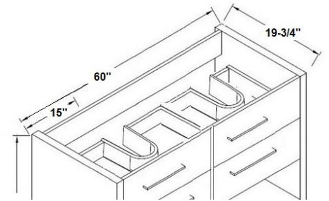
Intérieur / Inside
