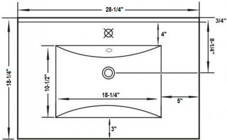
Trou de débordement Overflow hole
