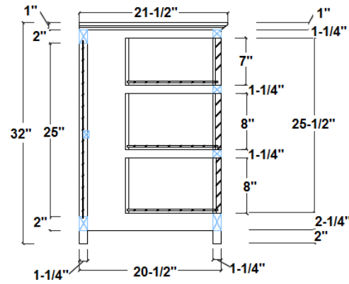
SIDES/COTES
