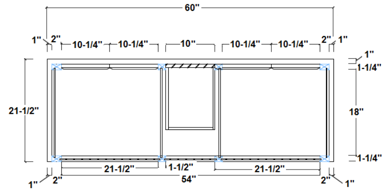
TOP/DESSUS
