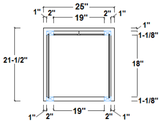
TOP/DESSUS
