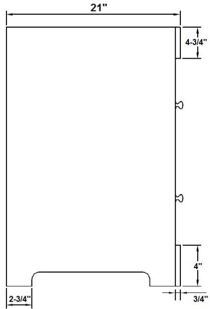
CÔTÉ / LEFT SIDE
